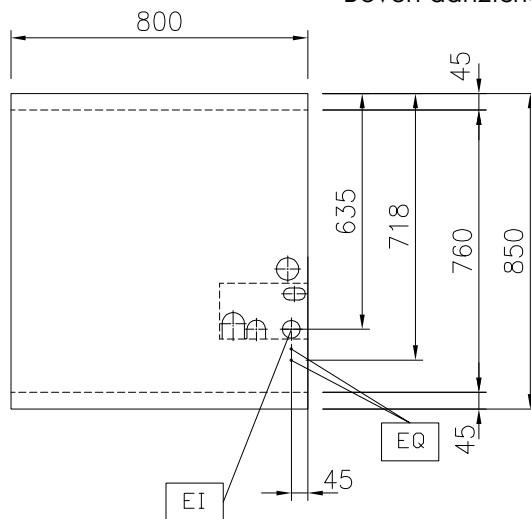
Boven aanzicht
