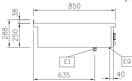
Zij aanzicht
