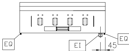
Front aanzicht
